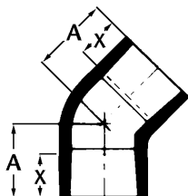
45° Elbow
