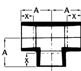
Tee
